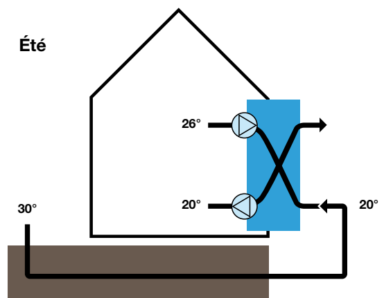
Principe de fonctionnement du puits canadien.
